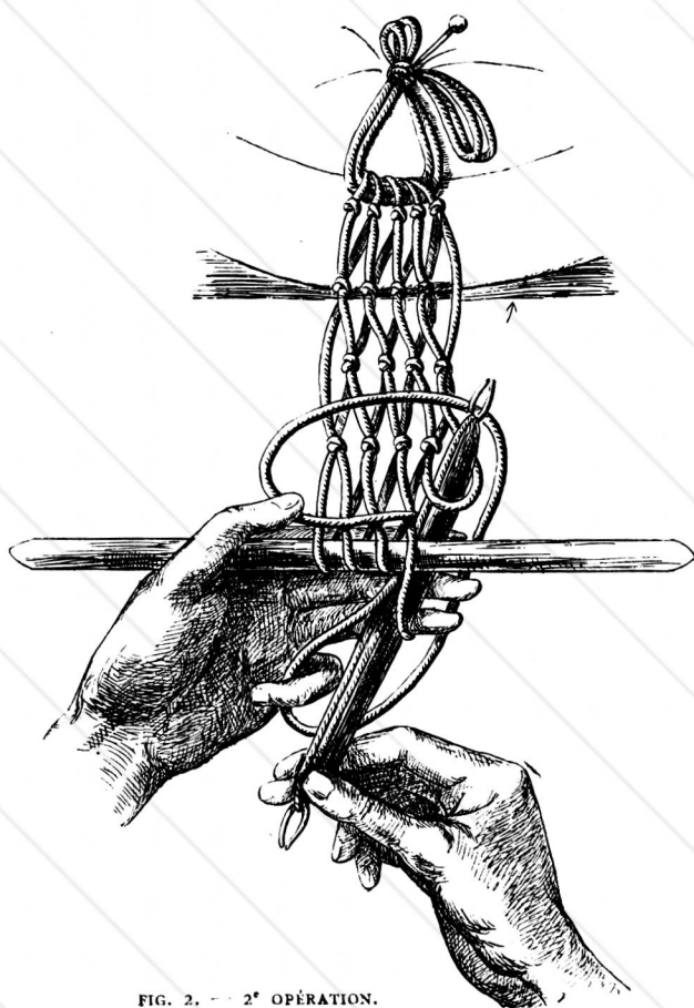
FIG. 2. — 2 e OPÉRATION.
